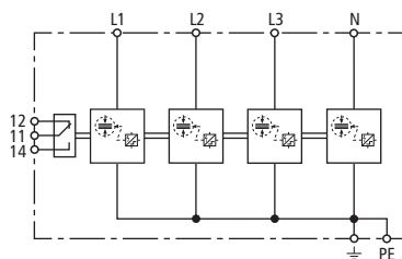
Schemat połączeń
