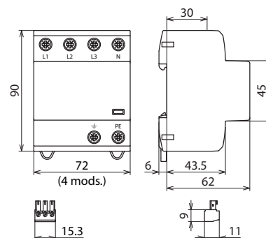
Rysunek wymiarowy
